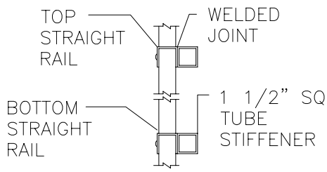
SECTION-A
